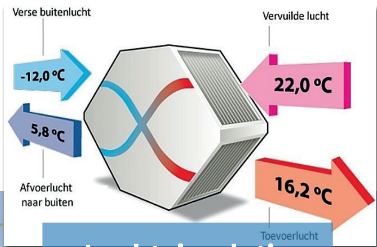
Luchtcirculatie
